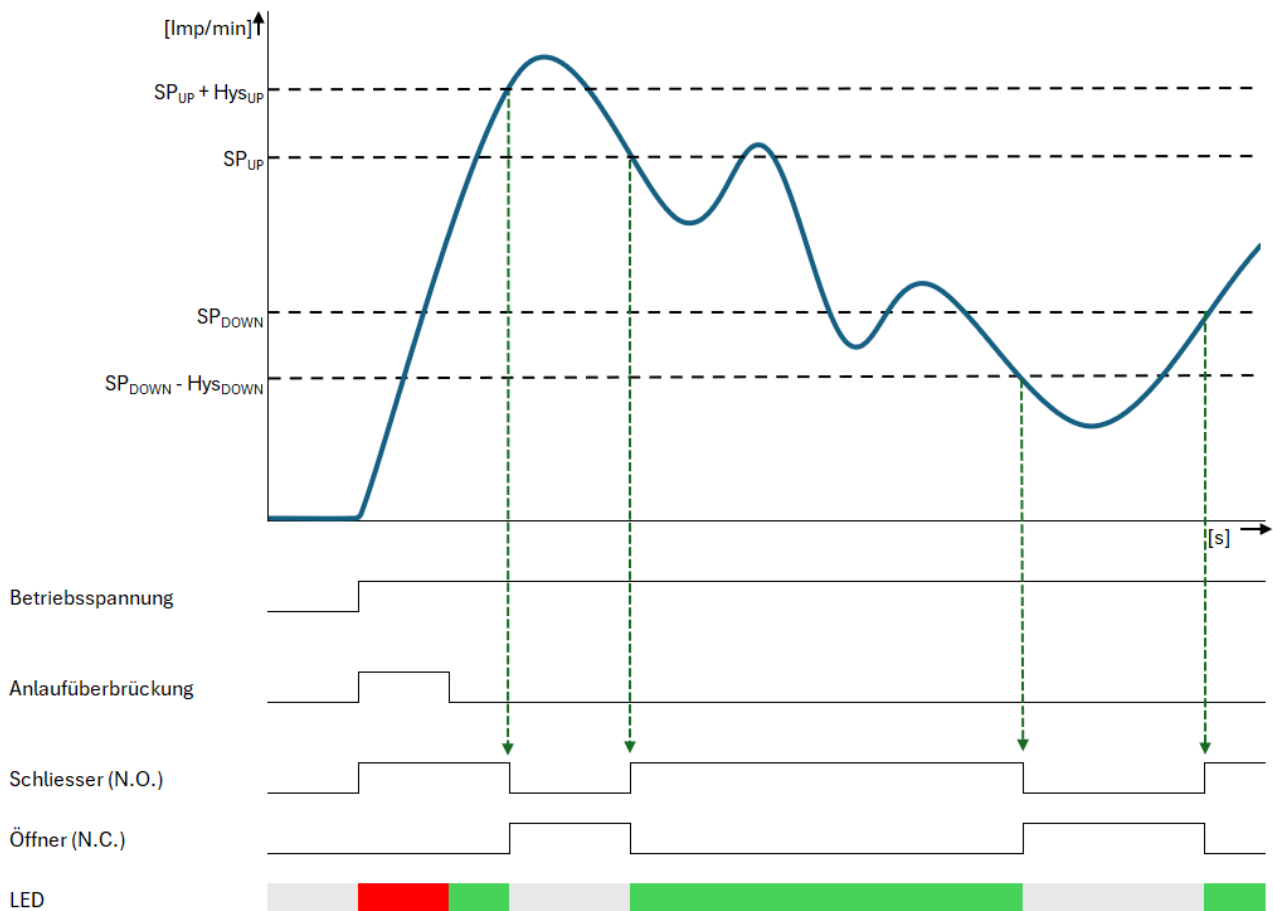
Funktionsdiagramm Drehzahlbereich
