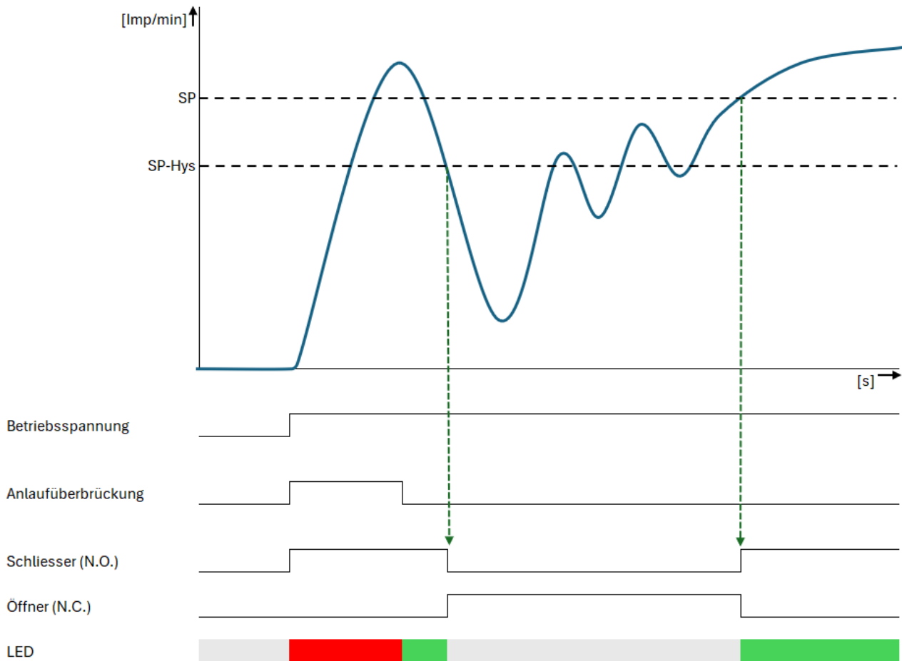
Funktionsdiagramm Solldrehzahl
